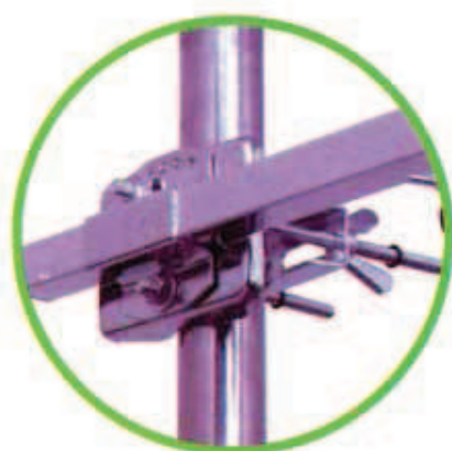
K593 - Staffa completa attacco per antenna
